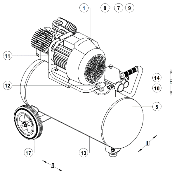
Рисунок 9 - Общий вид компрессора СБ4/С-50.Ј2047В
