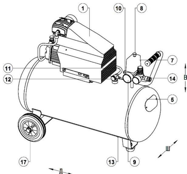
Рисунок 7 - Общий вид компрессора СБ4/С-50.Ј1047В, СБ4/С-50.Ј1048В
