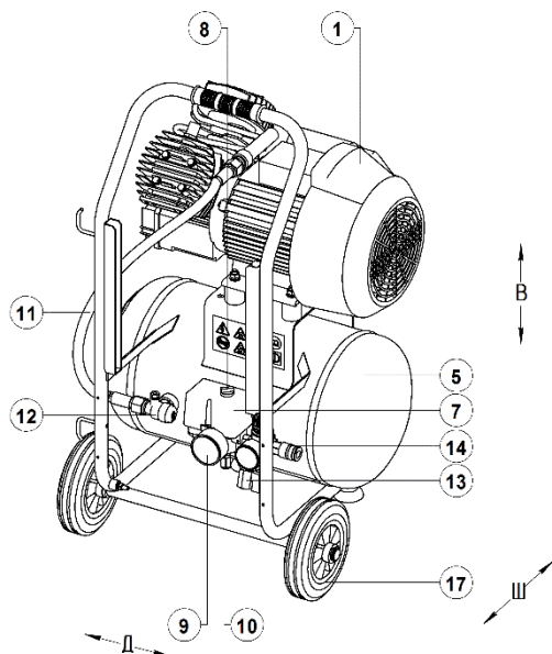
Рисунок 8 - Общий вид компрессора СБ4/С-20.Ј2047В
