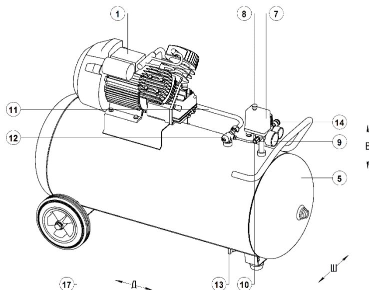
Рисунок 10 - Общий вид компрессора СБ4/С-100.J2047В
