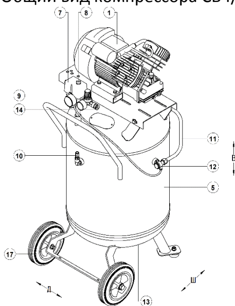
Рисунок 10 - Общий вид компрессора СБ4/С-100.J2047ВВ
