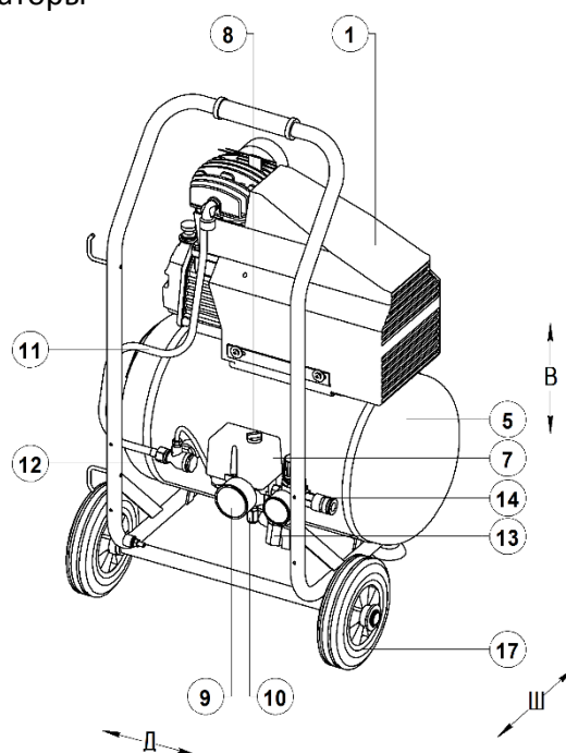
Рисунок 5 - Общий вид компрессора СБ4/С-20.Ј1047В, СБ4/С-20.Ј1048В
